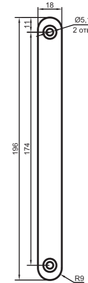
77772 Ответная планка BORDER МАГНИТ Черный
