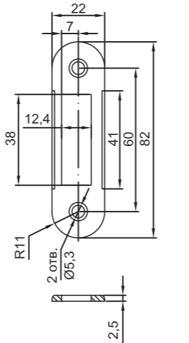
80128 Ответная планка BORDER 169.02 Белый
