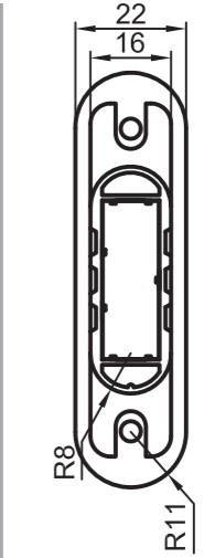
77772 Ответная планка BORDER МАГНИТ Черный
