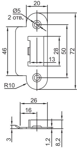
77765 Ответная планка BORDER 150 Белый
